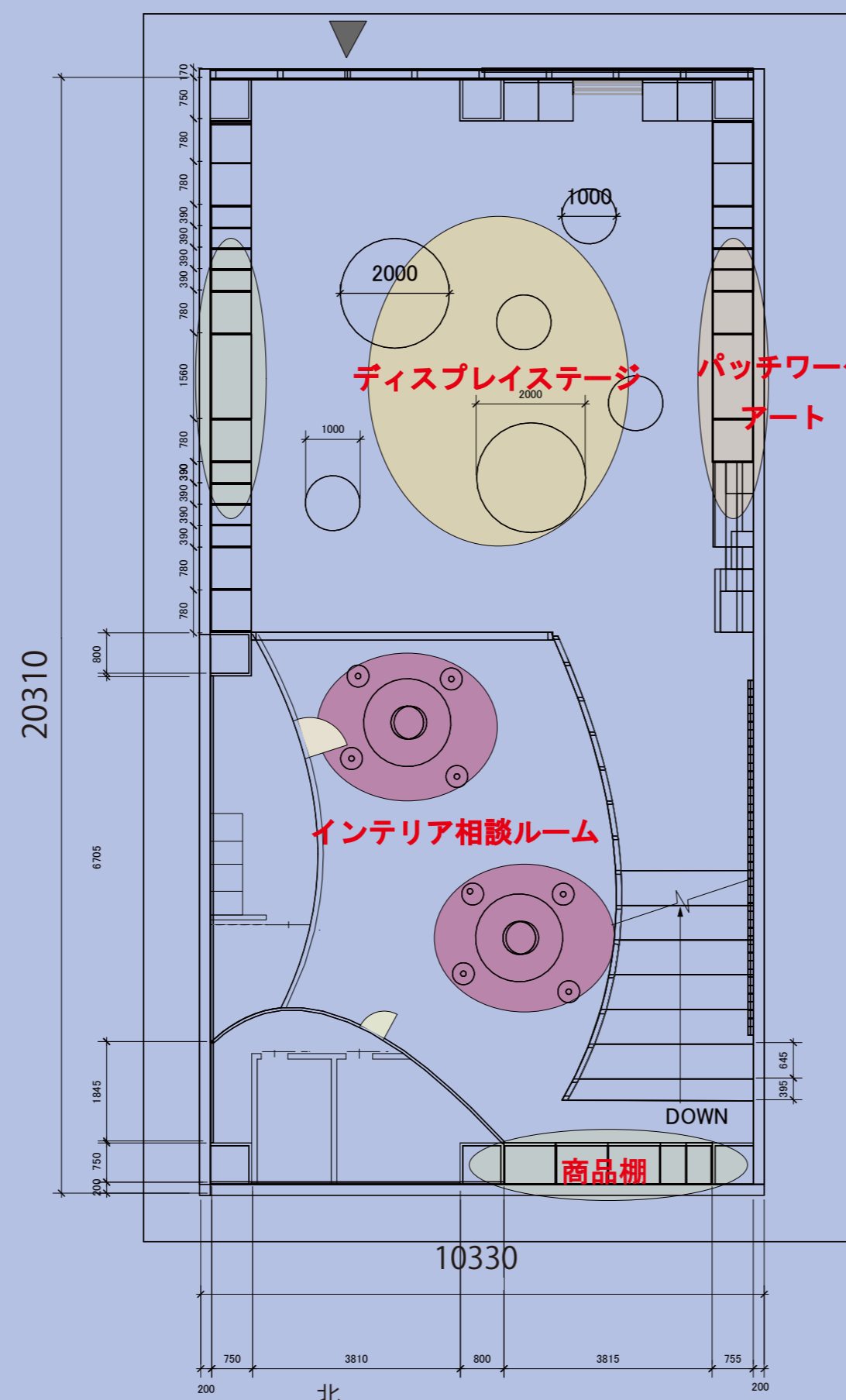
2階 平面図 S=1/50
