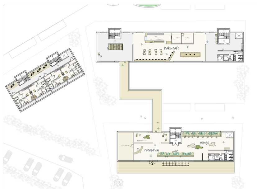
3F 平面図 1:400
