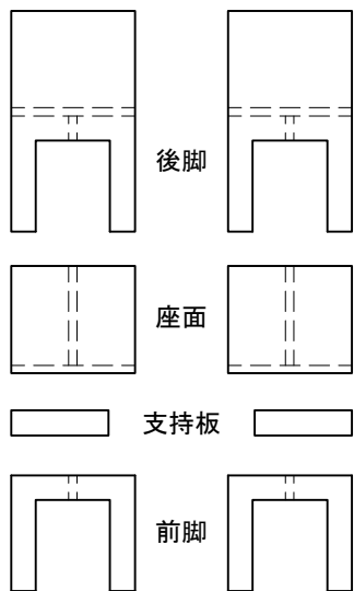
椅子(2脚) (奥行き420×幅450×高さ800) (座面高さ450)
